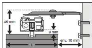
Pose avec équerre. Ecartement réglable : 60-108 mm. ( Accessoire spécial : 108-156 mm/156-204 mm. )
